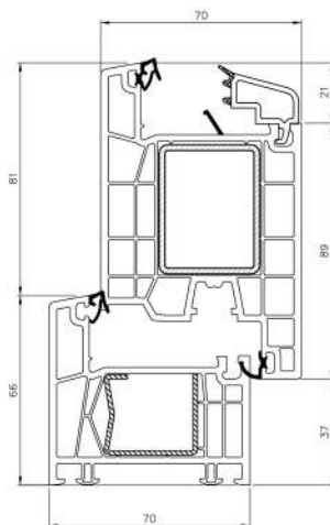
COMBINAZIONE ANTAFERMAVETRO MAGGIORATA TELAIO SU NUOVO
