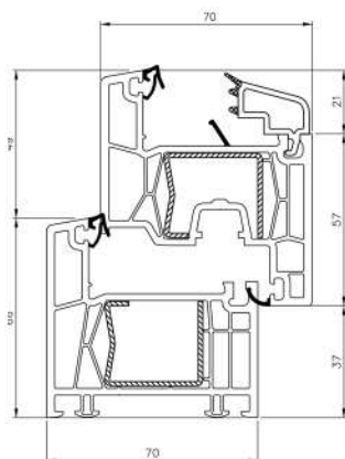
COMBINAZIONE ANTAFERMAVETRO TELAIO SU NUOVO
