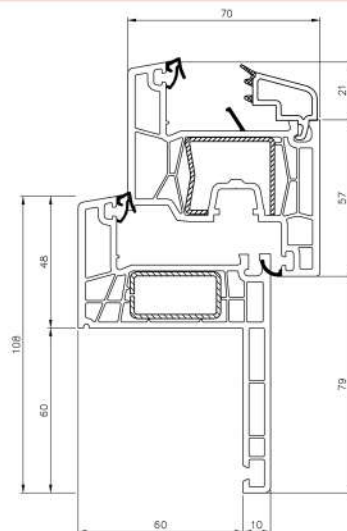
COMBINAZIONE ANTAFERMAVETRO TELAIO RINNOVO
