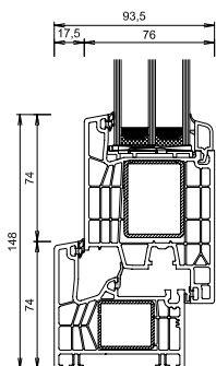
COMBINAZIONE ANTA MAGGIORATA-FERMAVETRO TELAIO SU NUOVO
