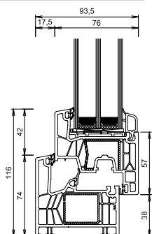
COMBINAZIONE ANTA-FERMAVETRO TELAIO SU NUOVO
