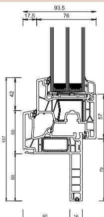
COMBINAZIONE ANTA-FERMAVETRO RINNOVO
