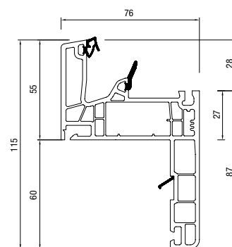
TELAIO RINNOVO DISPONIBILE DA NOVEMBRE 2015
